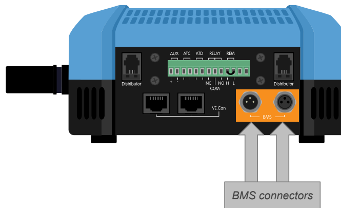
Placering av BMS-kabelkontakt
